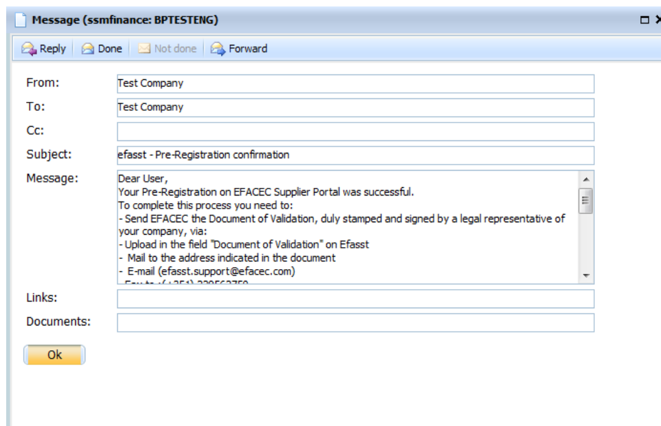
Fig. 22 - Message Detail
